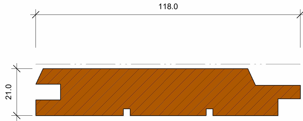
7205-1 TF TGV GLAT 25x125 1:1
