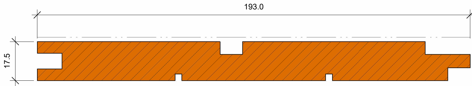
6613-1 CT GU-U GLAT 22X200 1:1
